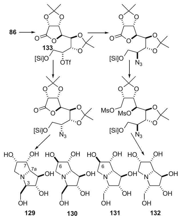
Scheme 26.
