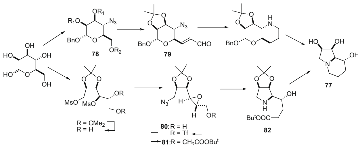
Scheme 16.
