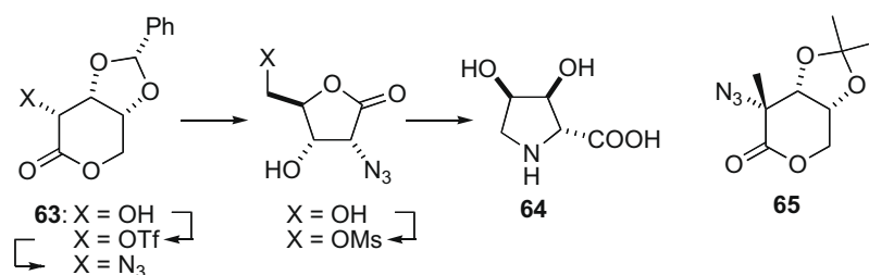
Scheme 14.
