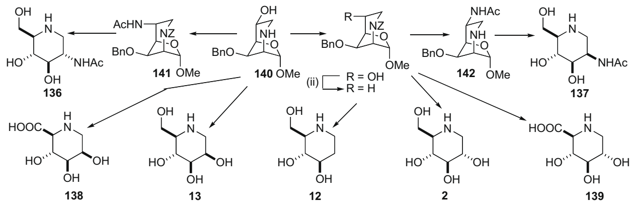
Scheme 28.
