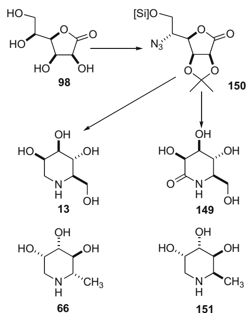
Scheme 31.
