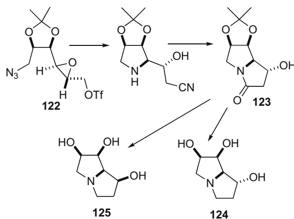
Scheme 24.
