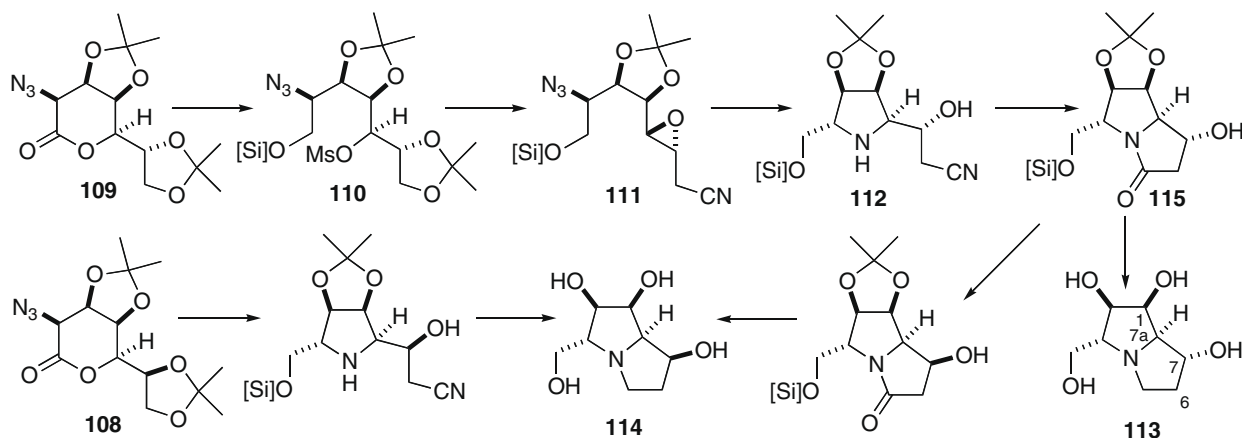
Scheme 21.
