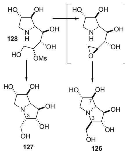
Scheme 25.
