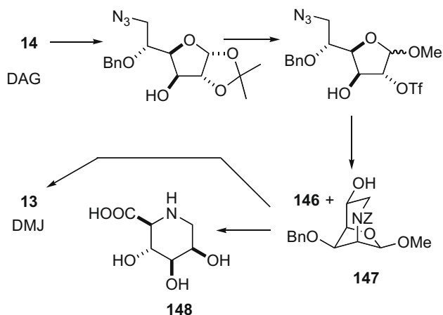
Scheme 30.
