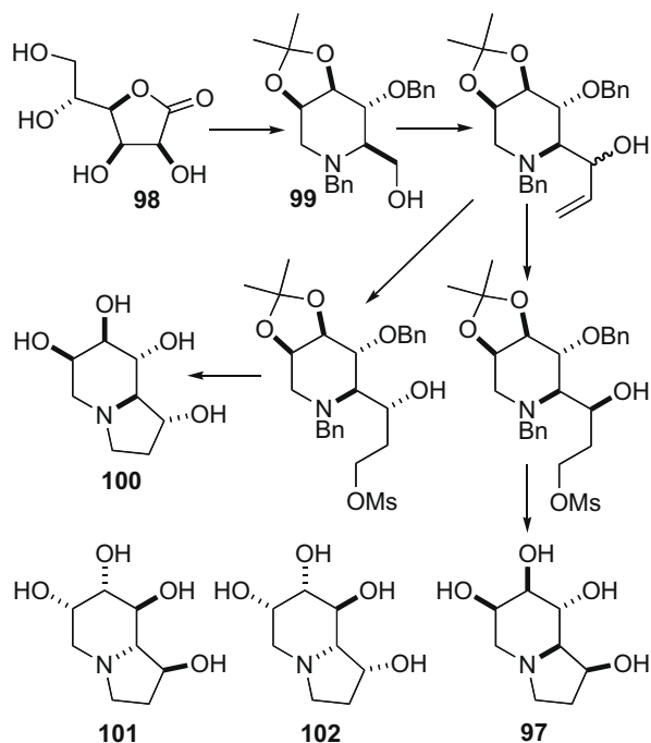
Scheme 19.
